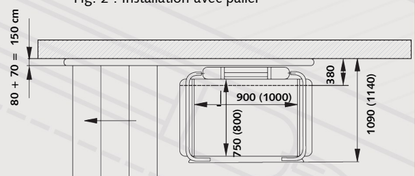
Fig. 2 : Installation avec palier
