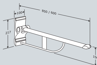
Dim. en position rabattue : 192 mm
