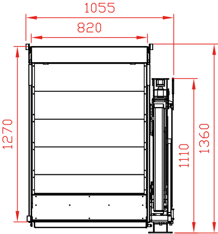
OWU006 en position de travail Montage côté gauche
