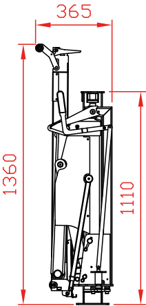
OWU006 en position route Montage côté droit
