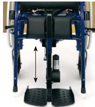
14.73HM Repose-pieds réglables électriques pour 18.64M.
