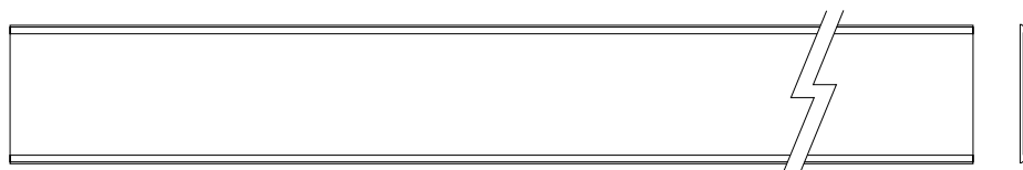
volea 100 w ... x h 114 x d 3 mm w ... x h 4,48 x d 0,11"
