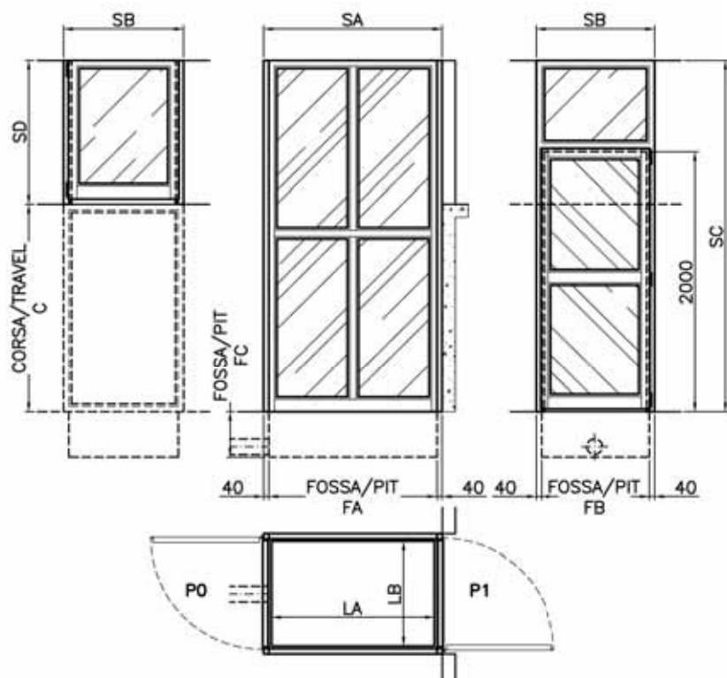
PLATE-FORME À SORTIES OPPOSÉES - SBARCHI CONTRAPPOSTI
