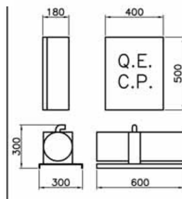
DIMENSIONE CENTRALINA E QUADRO DIMENSION DE CENTRALE ÉLECTRO HYDRAULIQUE ET PANNEAU ÉLECTRIQUE
